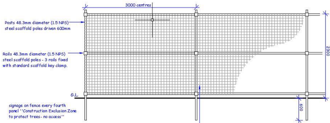
ELEVATION 1:25
