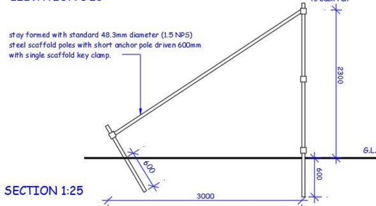
ELEVATION 1:25
