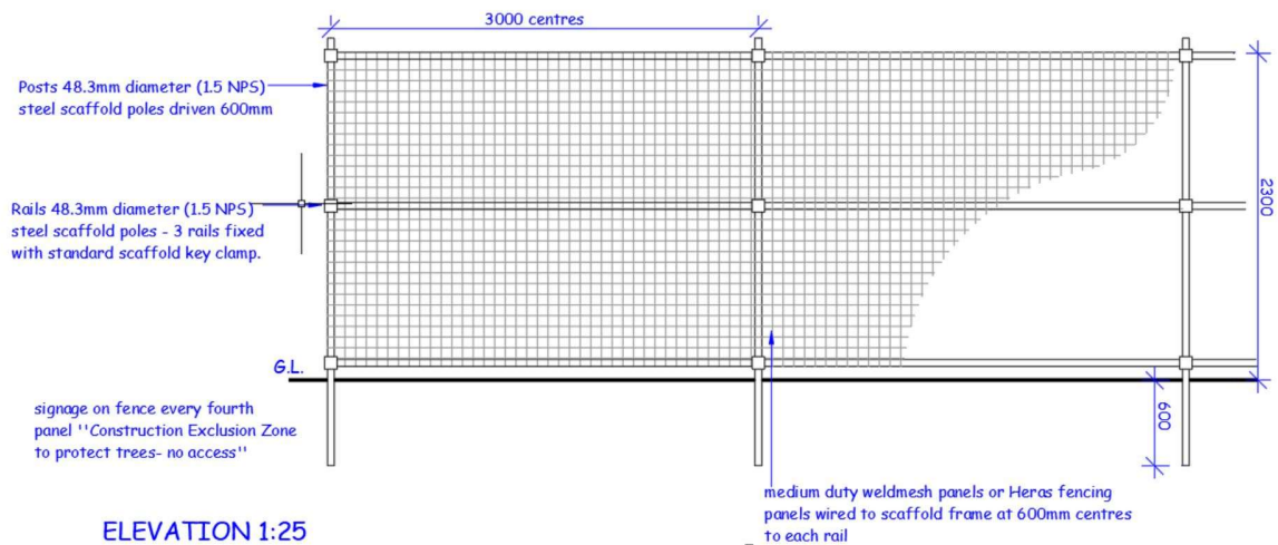
ELEVATION 1:25
