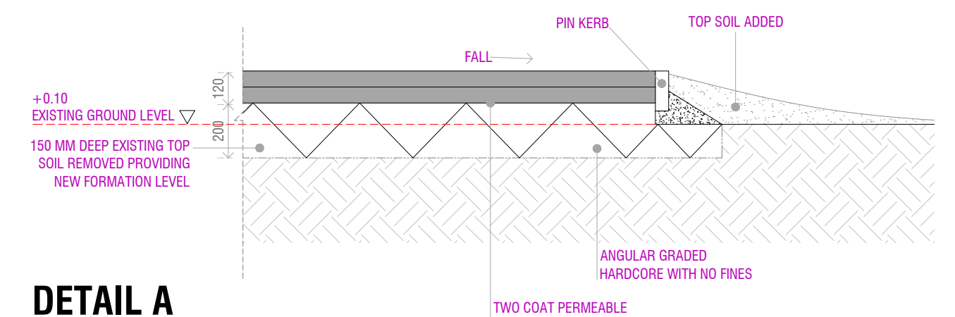
Scale: 1:20@ A1
