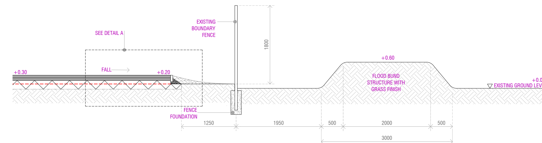
Scale: 1:50@A1
