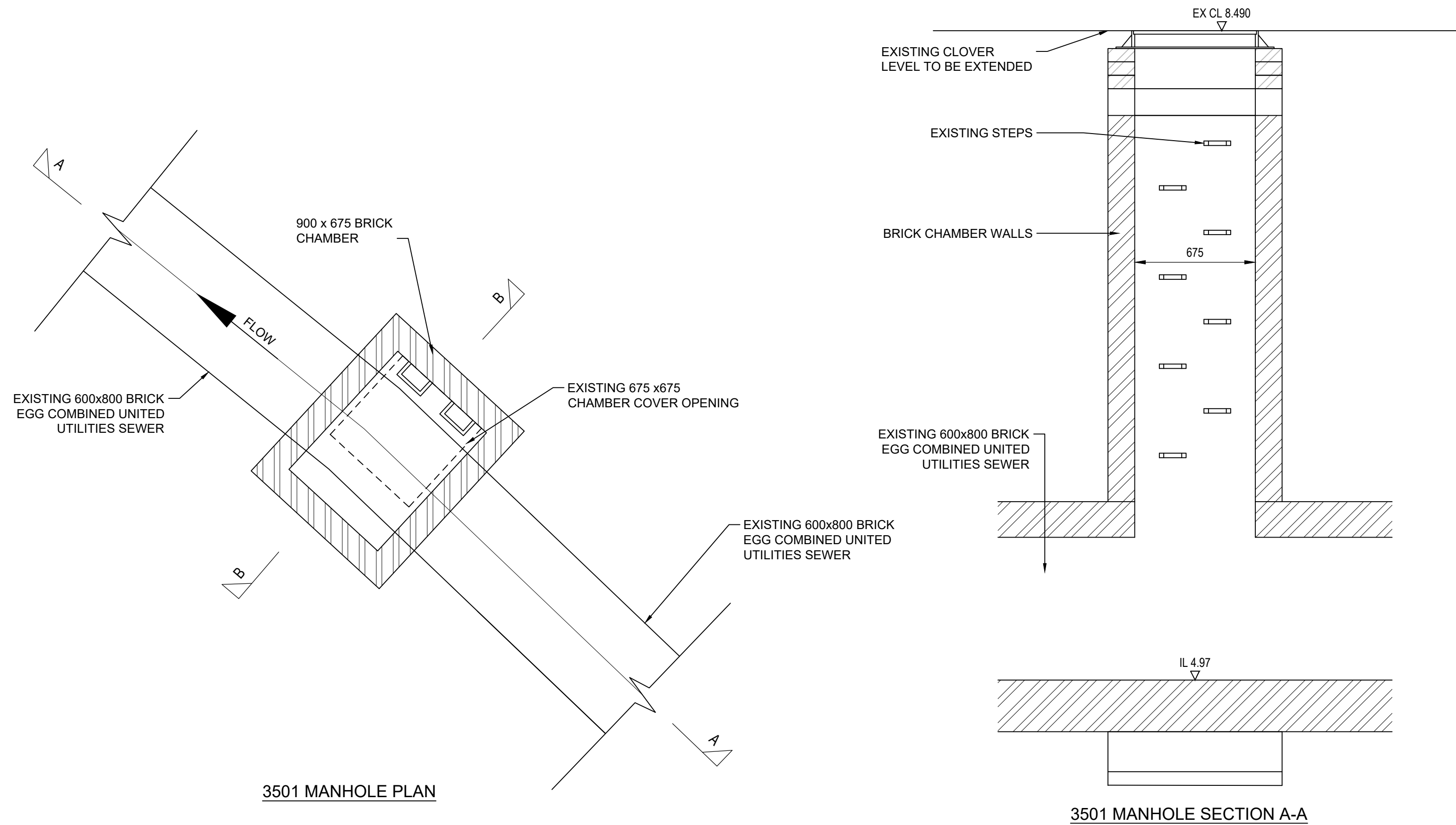
3501 MANHOLE SECTION A-A
