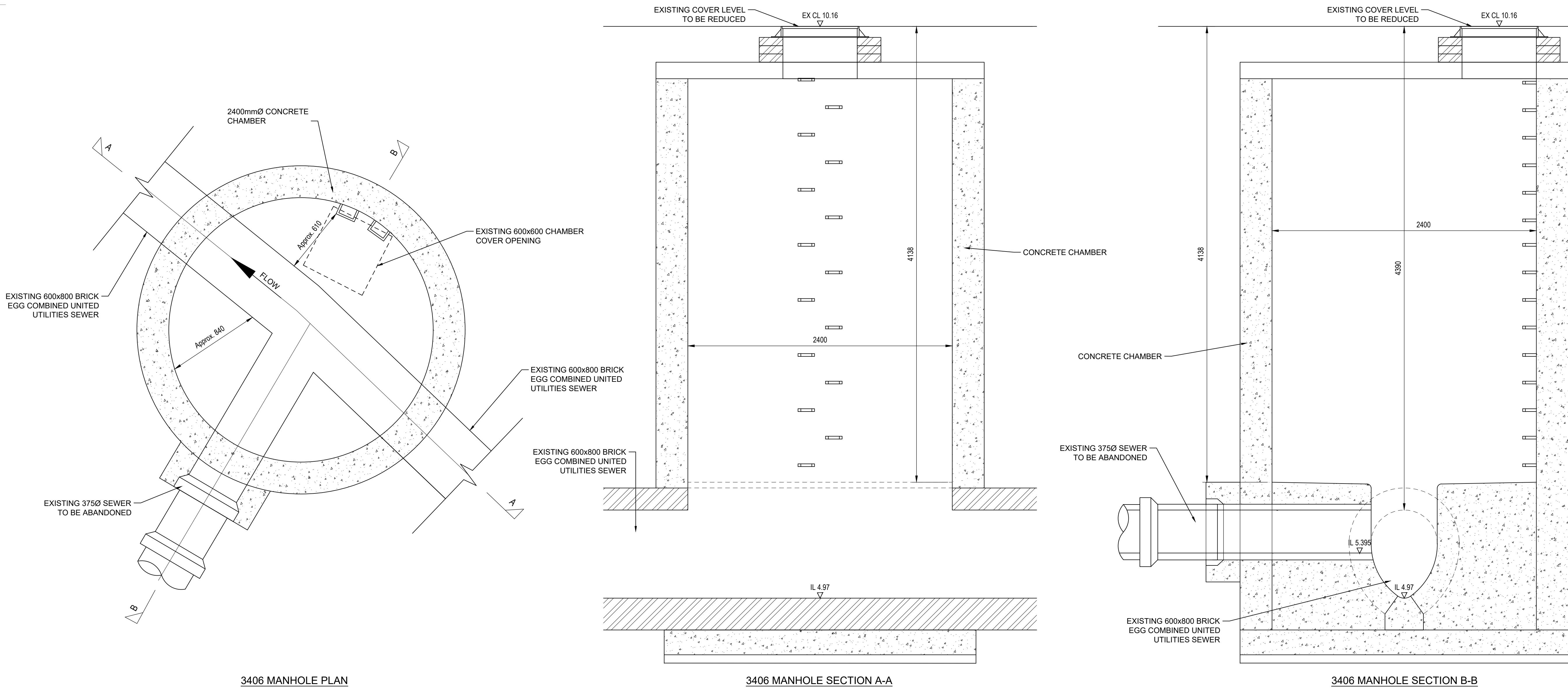
3406 MANHOLE PLAN
