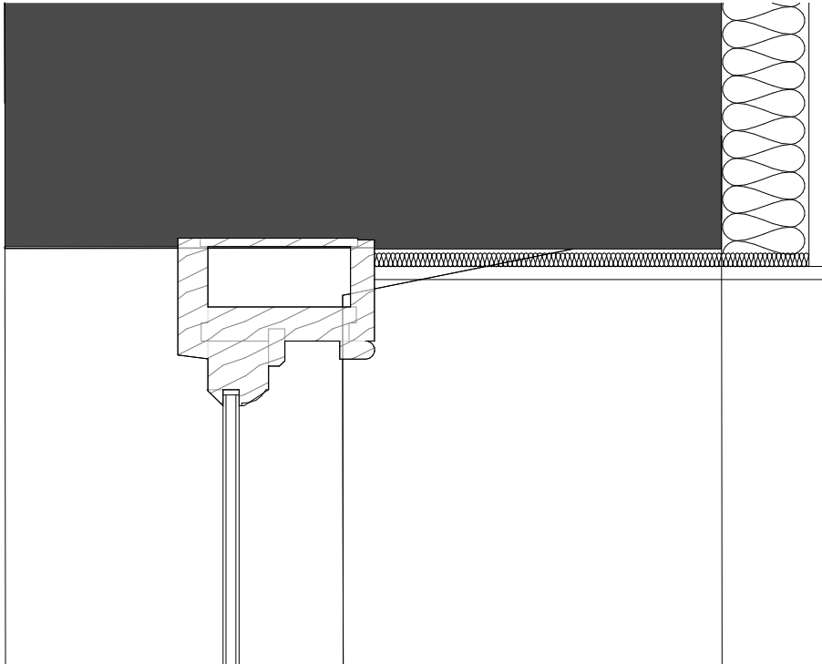
Jamb Detail ZZ-DR-A-31309 SCALE: 1 : 5
