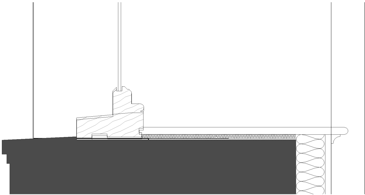
Cill Detail ZZ-DR-A-31309 SCALE: 1 : 5
