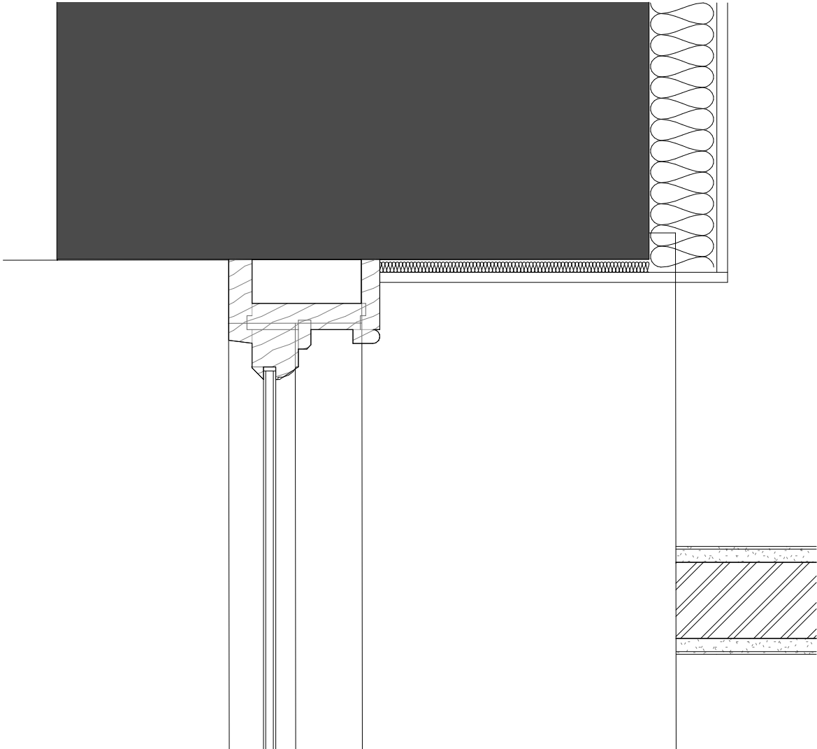
Jamb Detail ZZ-DR-A-31308 SCALE: 1 : 5
