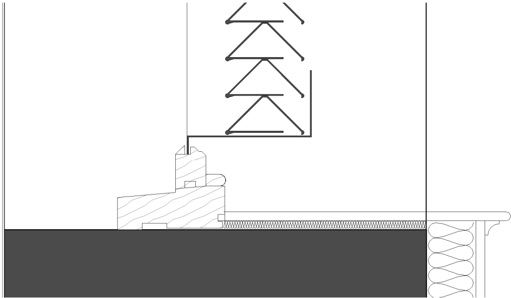
Cill detail ZZ-DR-A-31308 SCALE: 1 : 5
