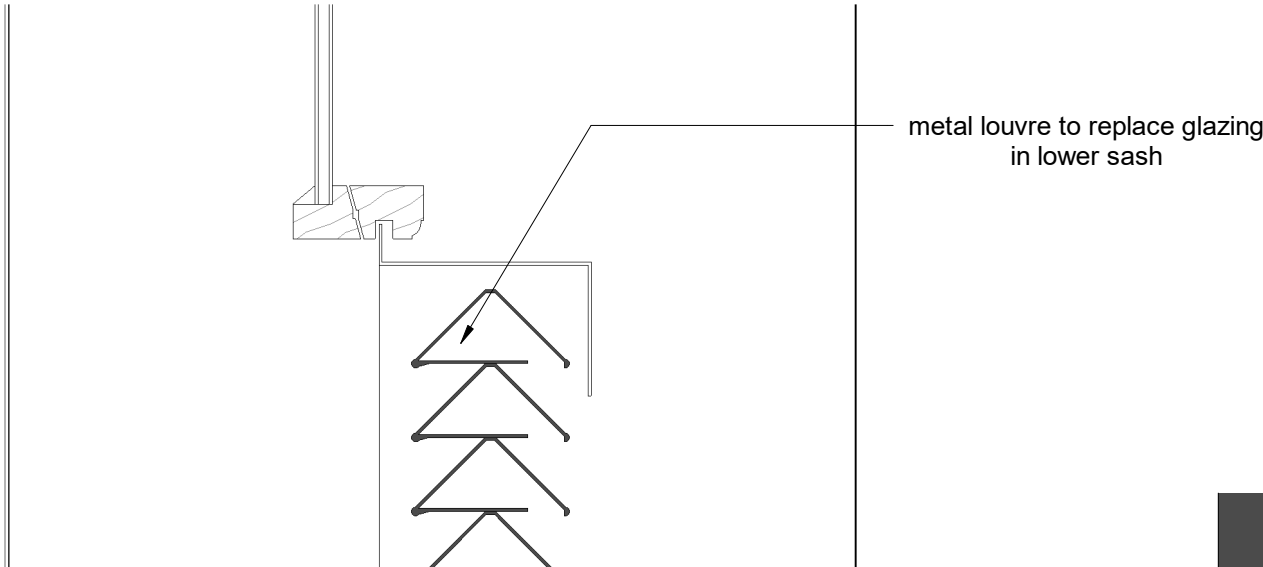
Louver detail ZZ-DR-A-31308 SCALE: 1 : 5
