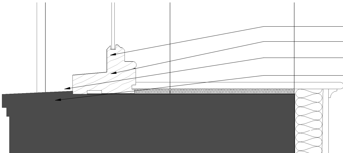
Cill detail ZZ-DR-A-31307 SCALE: 1 : 5
