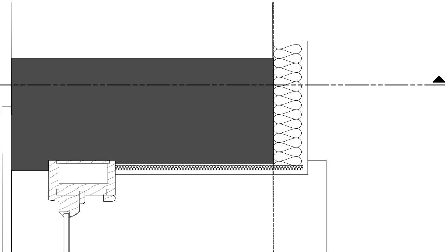
Jamb detail ZZ-DR-A-31307 SCALE: 1 : 5
