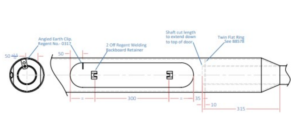
Door Detail
