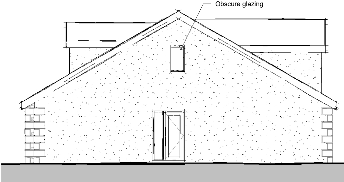
Side Elevation 01 1 : 100
