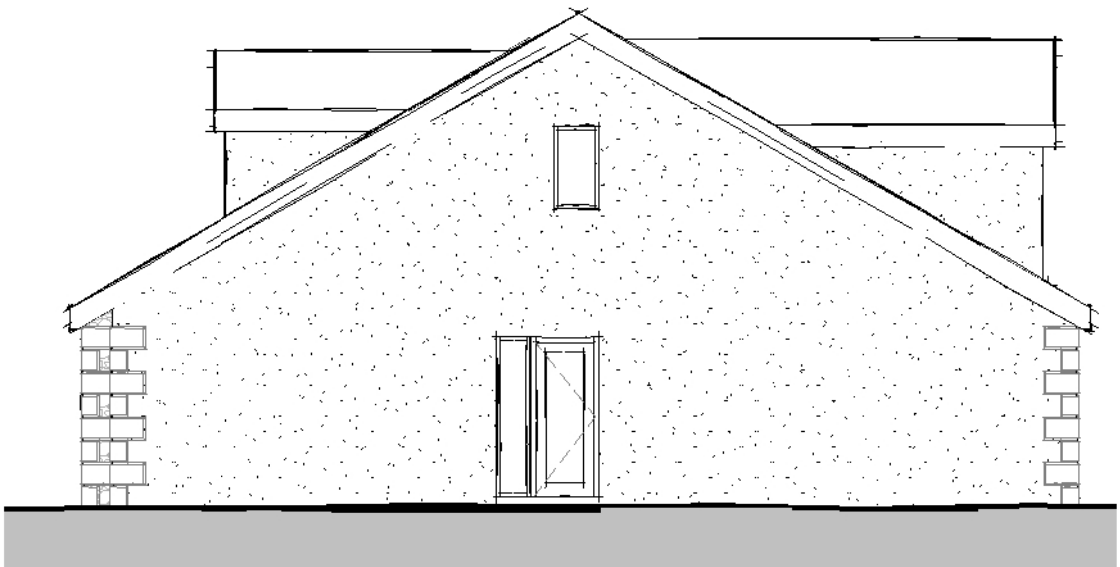
Side Elevation 01 1 : 100
